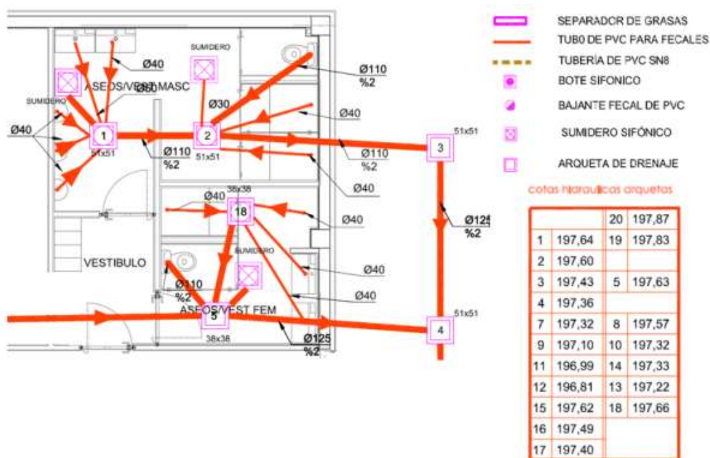
Imagen 10. Plano con la distribución de las redes de fontanería y saneamiento en los aseos y vestuarios.
