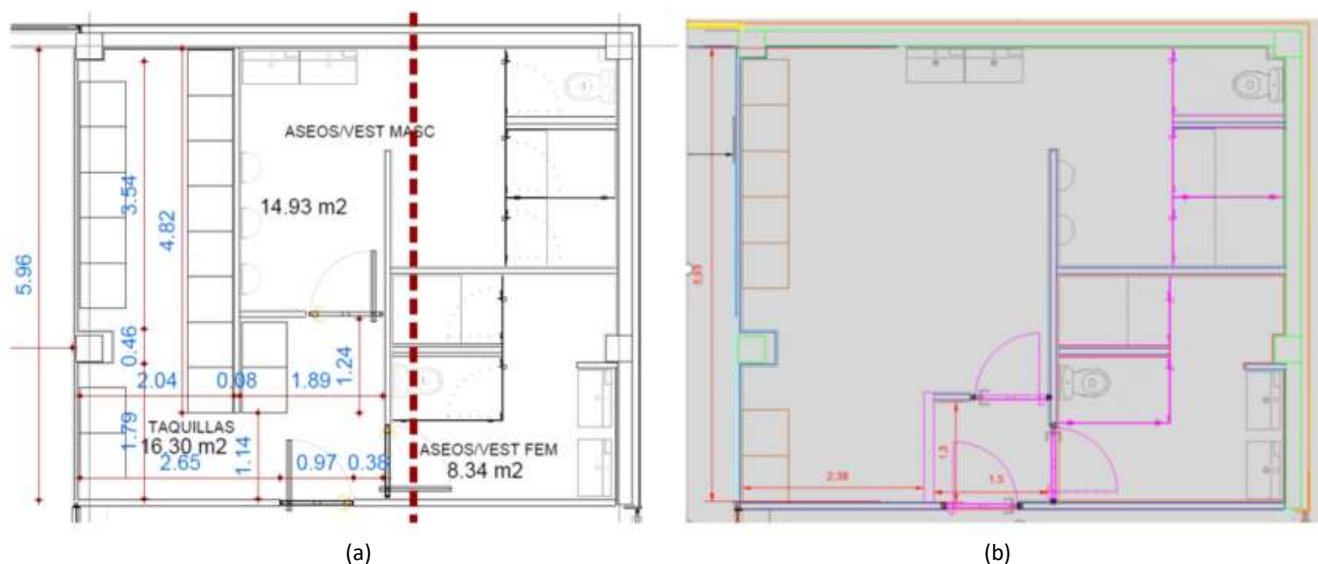
Imagen 1. Comparativa del estado actual y futuro de los aseos y vestuarios del parque de bomberos. (a) Estado actual de los vestuarios y aseos. (b) Propuesta de reforma con nueva distribución.
