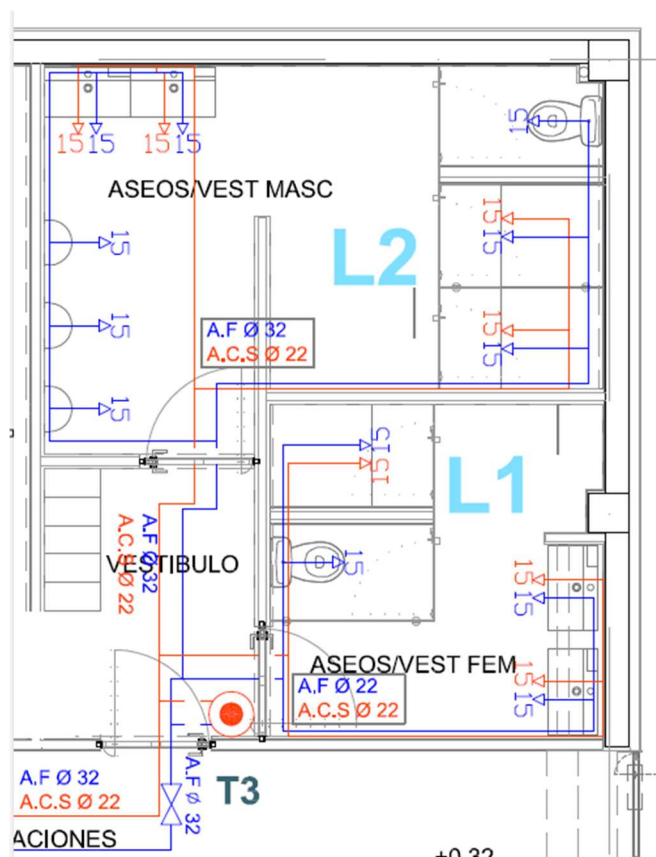
Imagen 9. Plano con la distribución de las redes de fontanería y saneamiento en los aseos y vestuarios.
